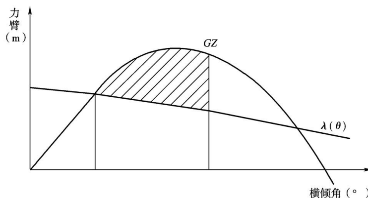
图 15.3.5.4 (5) ① 帆船稳性曲线
